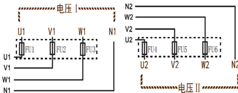
图10-4 GSTS60-ZG端子接线说明
