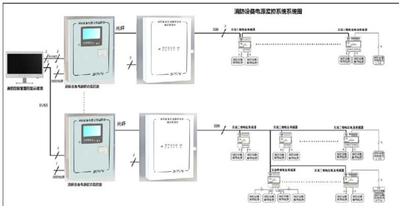
图2-1 系统图
