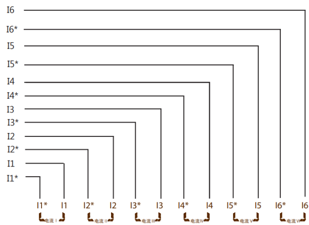
图10-14 GSTD06-ZG 端子接线说明
