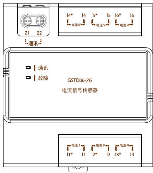
图10-13 GSTD06-ZG电流信号传感器
