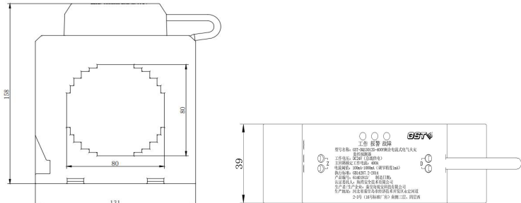
图 1 外观结构尺寸
