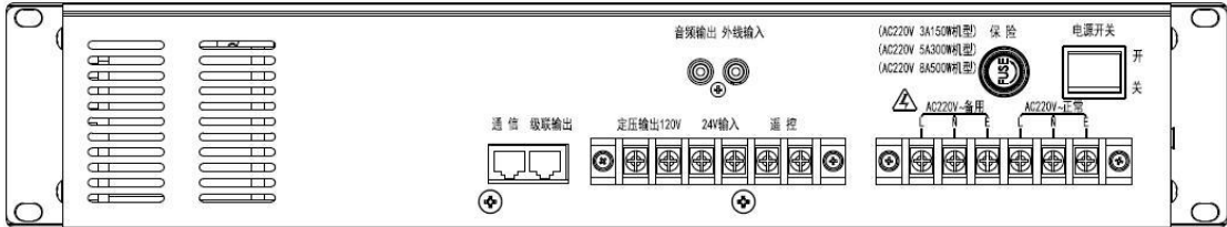
图 2.2.1 LT6242/300 接线端子说明表
