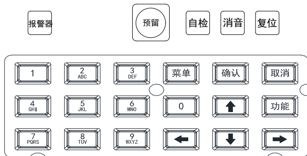
图 4-1 按键面板
