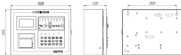
图 2-1 外观示意图
