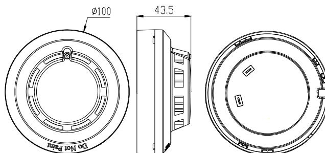
图 1 探测器外形示意图
