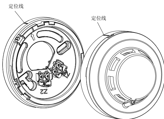
图4 探测器与底座安装示意图
