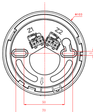
图3 探测器底座(DZ-07)外形示意图
